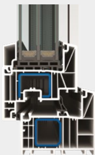
Uzavretá oceľová výstuha v ráme a oceľová výstuha krídla
