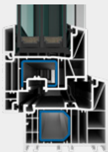
Uzavretá oceľová výstuha v ráme a oceľová výstuha krídla
